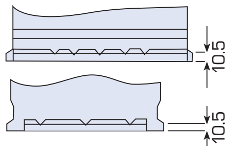
Bodenleiste B13
