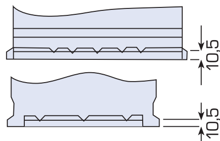
Bodenleiste B13
