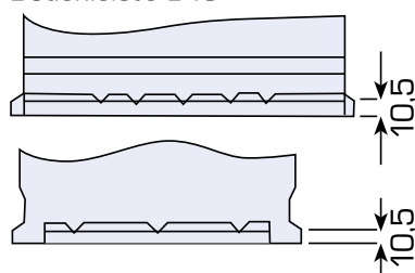
Bodenleiste B13
